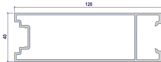
AE400 120mm Stile
